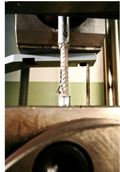
Prüfung von Betonstahl
