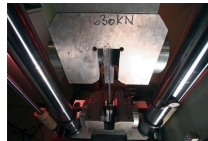
Prüfung von Spannstahl
