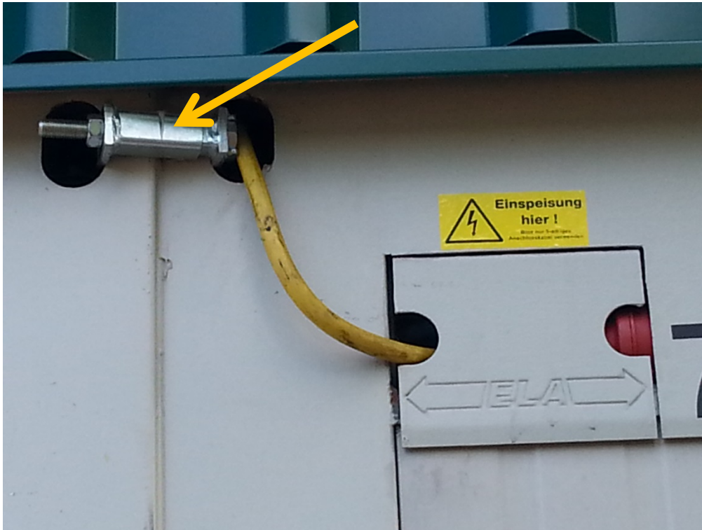
Bild 5: Elektroverbindung zwischen Containermodulen
