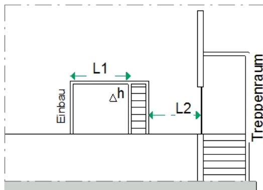
Schnitt
