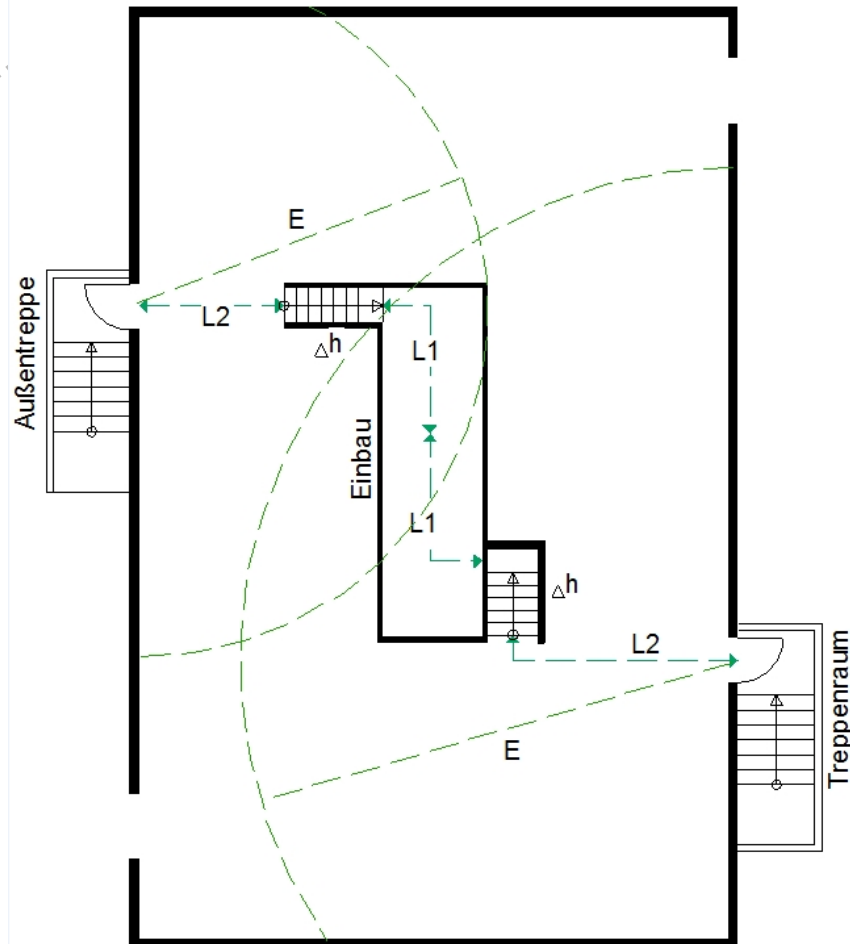
Grundriss
