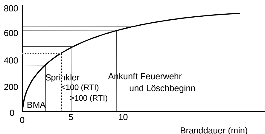
Abb. 3: Reaktionszeiten: Sprinkler im Vergleich zu automatischen Brandmeldeanlagen und der Feuerwehr
