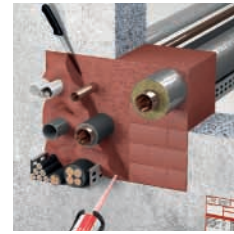
Kombiabschottungen ZZ-Brandschutzschaum 2K NE
