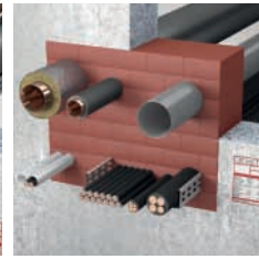
Kombiabschottungen ZZ-Steine 200 BDS-N
